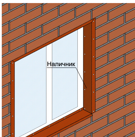
Рис. 29. Внешний вид оконного проёма с наличником с посыпкой (тип 4, таблица №2).
