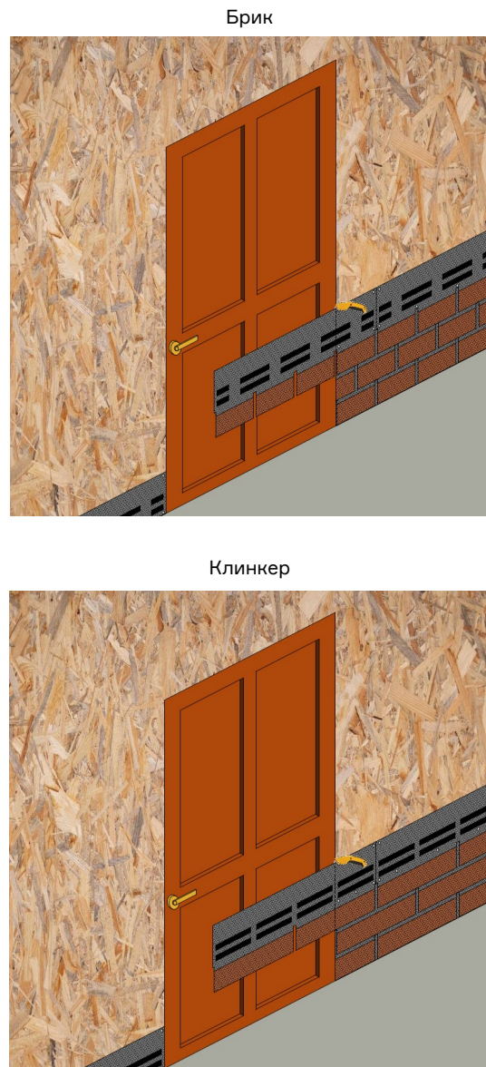
Рис. 35. Монтаж фасадной плитки вокруг дверного проёма.
