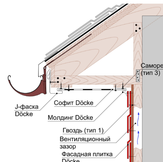
Рис. 37. Примыкание фасадной плитки к карнизному свесу.
