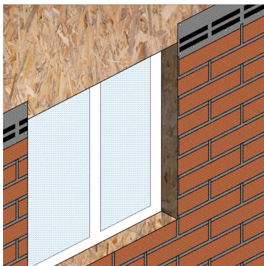
Рис. 26. Монтаж фасадной плитки вокруг оконного проёма.
