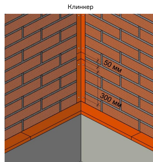
Рис. 23. Устройство внутренних углов при помощи металлических уголков с посыпкой.
