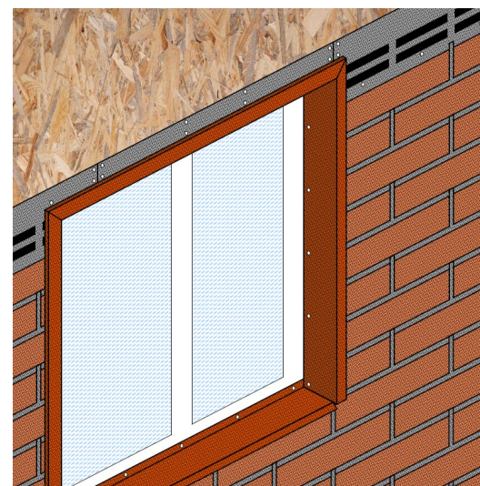
Рис. 33. Монтаж фасадной плитки над окном на наличник 3D с посыпкой (тип 5, таблица №2).
