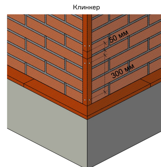
Рис. 16. Устройство внешних углов при помощи металлических уголков с посыпкой.
