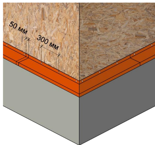
Рис. 6. Крепление металлических отливов с посыпкой.
