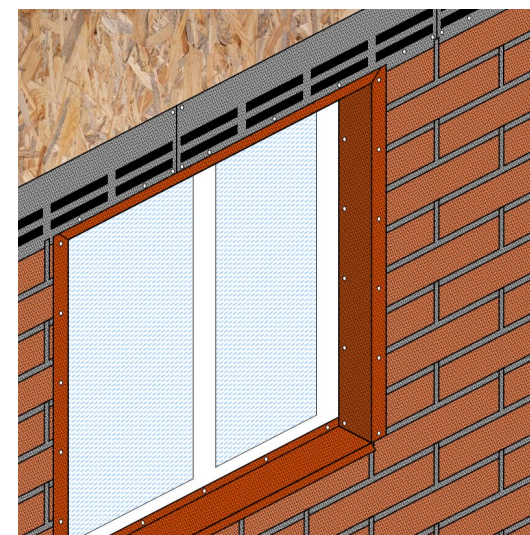
Рис. 28. Монтаж фасадной плитки над оконным проёмом.
