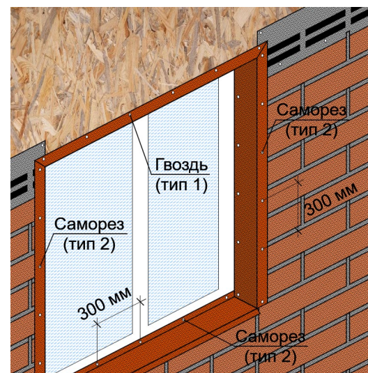
Рис. 27. Крепление металлических наличников с посыпкой.
