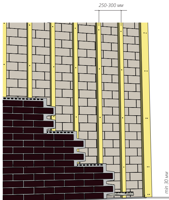
Рисунок 16. Деревянная обрешетка
