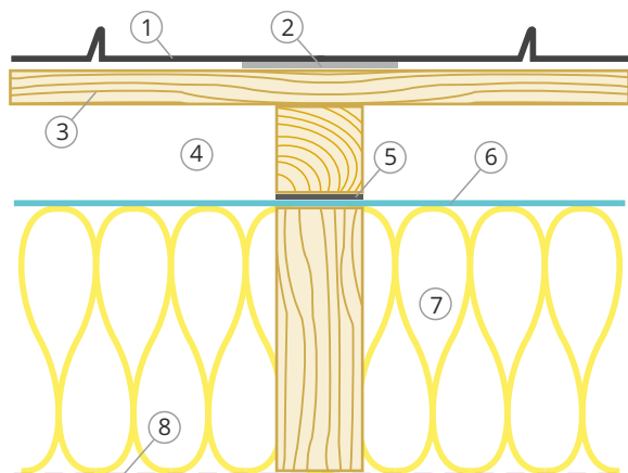
Разрезанная обрешетка
