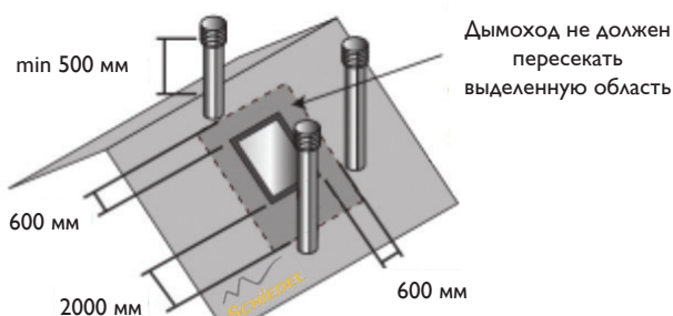
Рисунок 1 – схема расположения дымохода относительно мансардного окна
