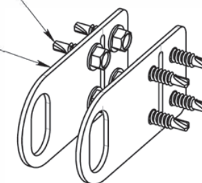
Проушина (в сборе)
